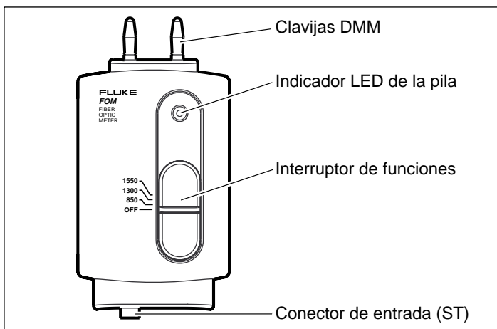
Figura 1. Medidor de potencia de fibras ópticas
