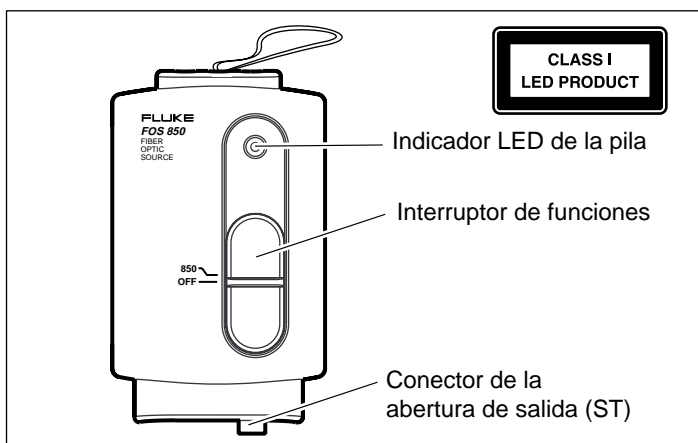
Figura 2. Fuente luminosa de fibras ópticas (se muestra la fuente 850)
