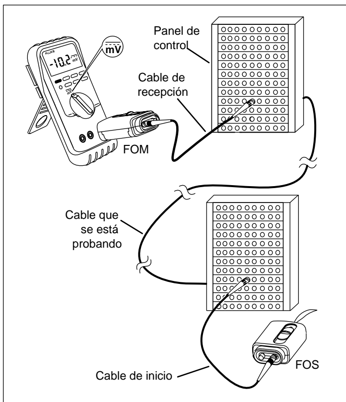
Figura 4. Medición de la pérdida óptica
