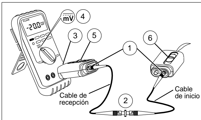
Figura 3. Medición de la salida para la referencia de la fuente
